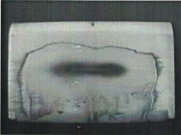
未加剂汽油沉积板
